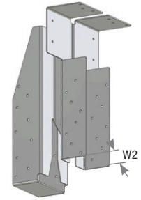
FWHBP Stud Pack Width
