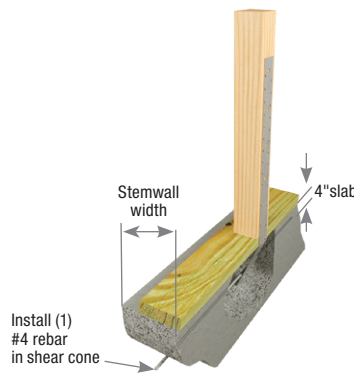
Typical HPAHD22-2P double pour edge installation
