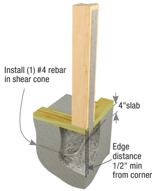
Typical HPAHD22-2P double pour corner installation
